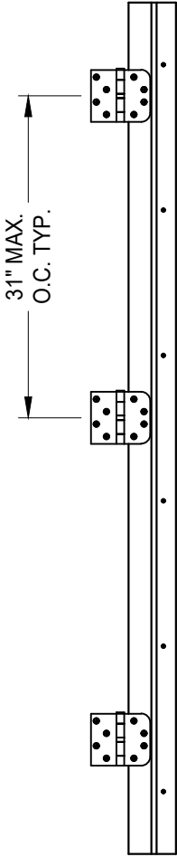
HINGE JAMB
